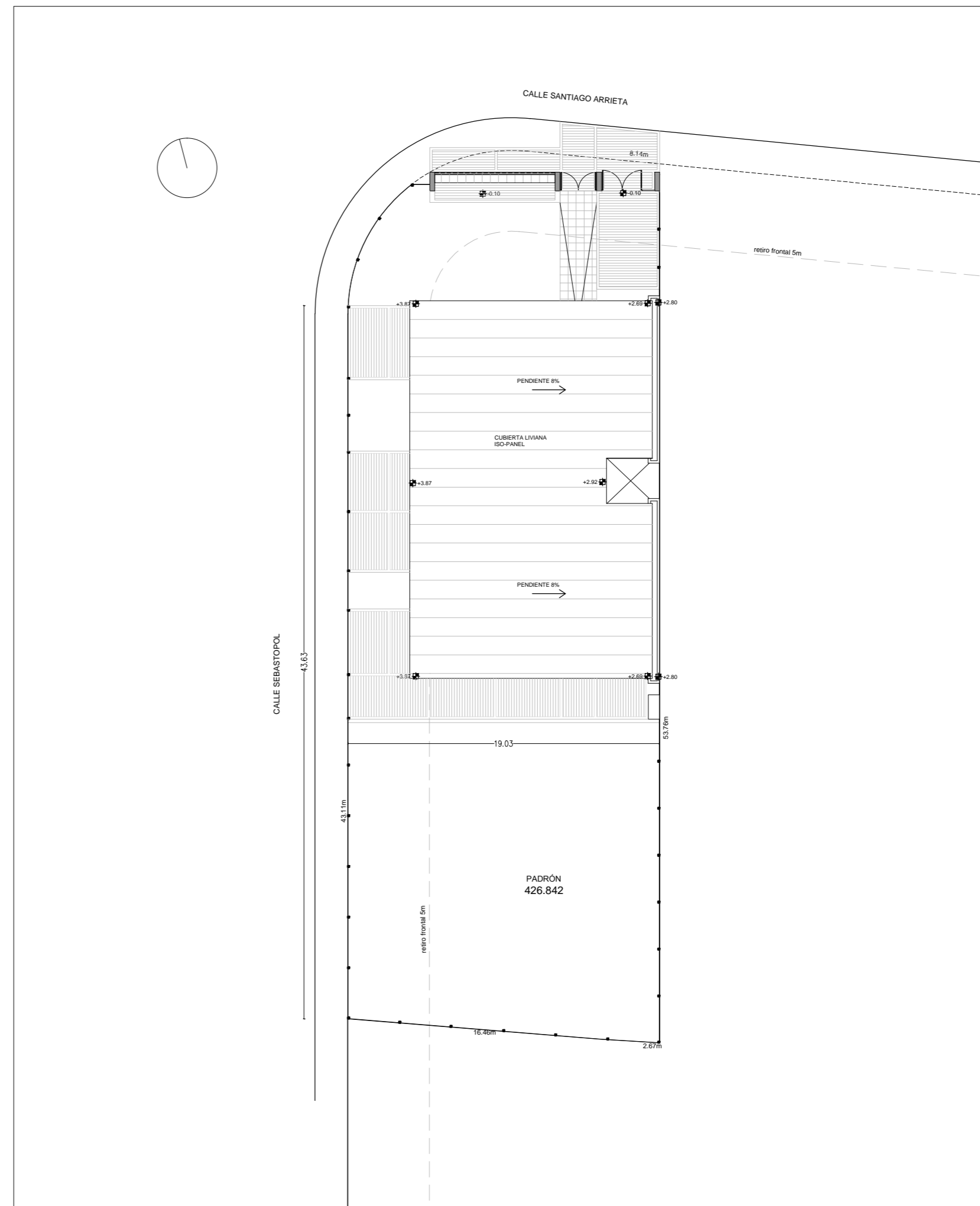
PLANTA UBICACIÓN ESC: 1:250
