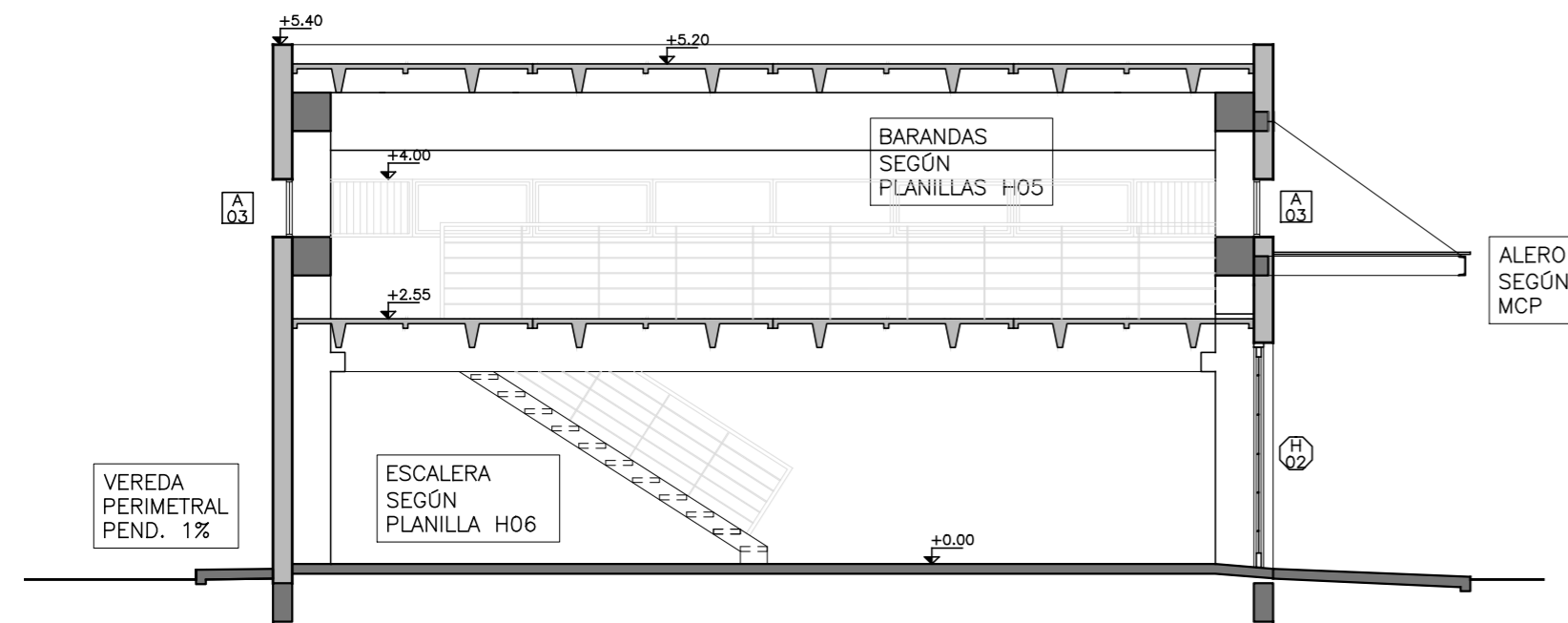
CORTE B ESC. 1.75
