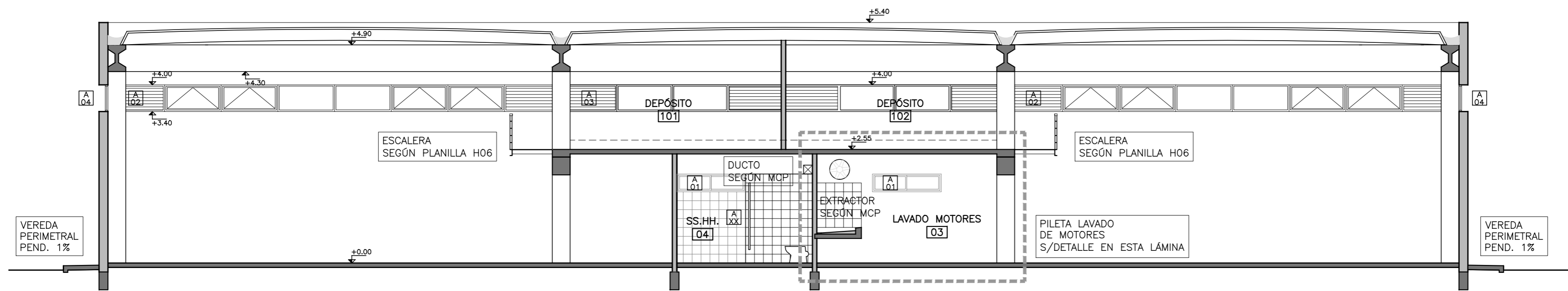
CORTE A ESC. 1.75
