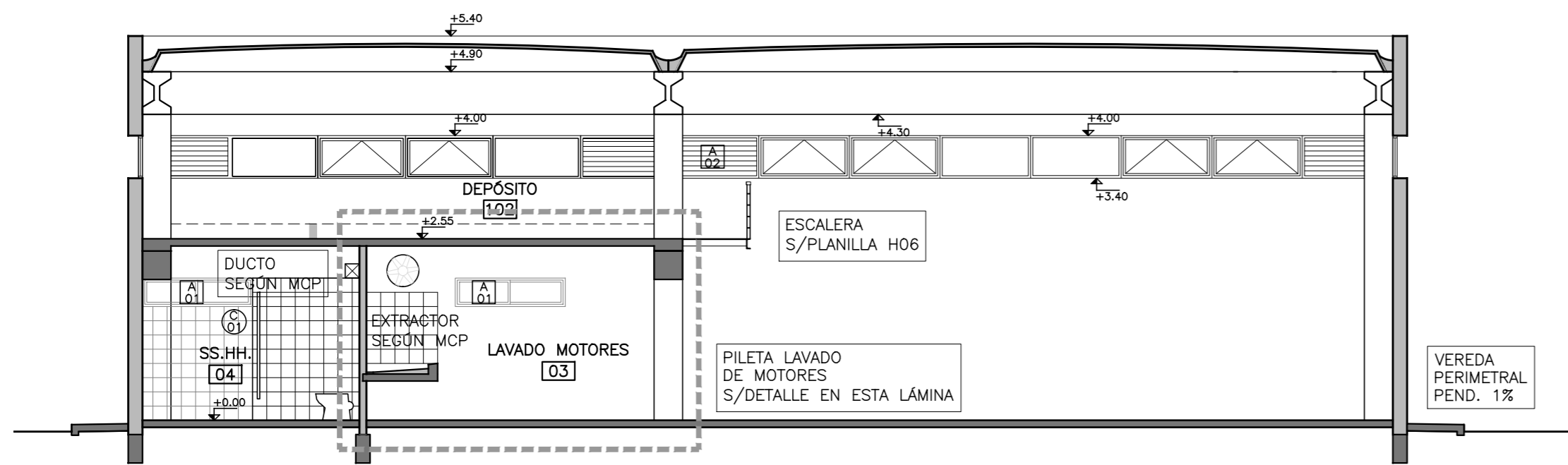
CORTE A ESC. 1.75
