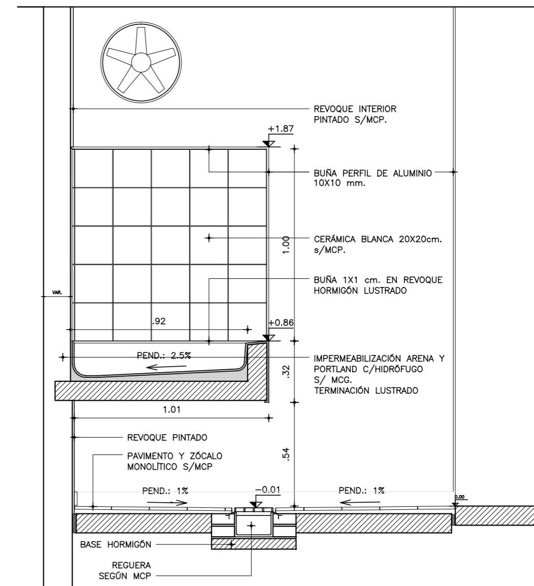
DETALLE GENÉRICO PILETA LAVADO DE MOTORES ESC. 1.20
